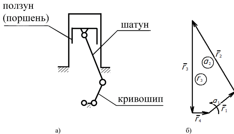
Рис. 1.1. Структурная схема механизма(а) и его векторная модель(б)
